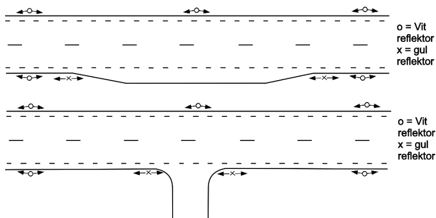
Figur 5. Placering av kantstolpar vid rast-, parkerings- och busshållplats (ovan) respektive korsning (nedan). Pilarna visar retroreflektorernas riktning.
