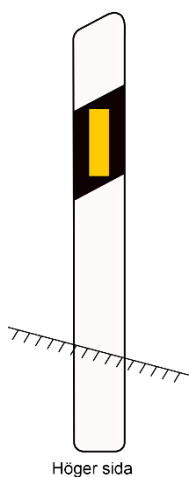
Figur 6. Utseende på kantstolpe, till höger i vägens färdriktning, direkt före respektive efter rast- parkerings- och busshållplats samt korsning och anslutning.
