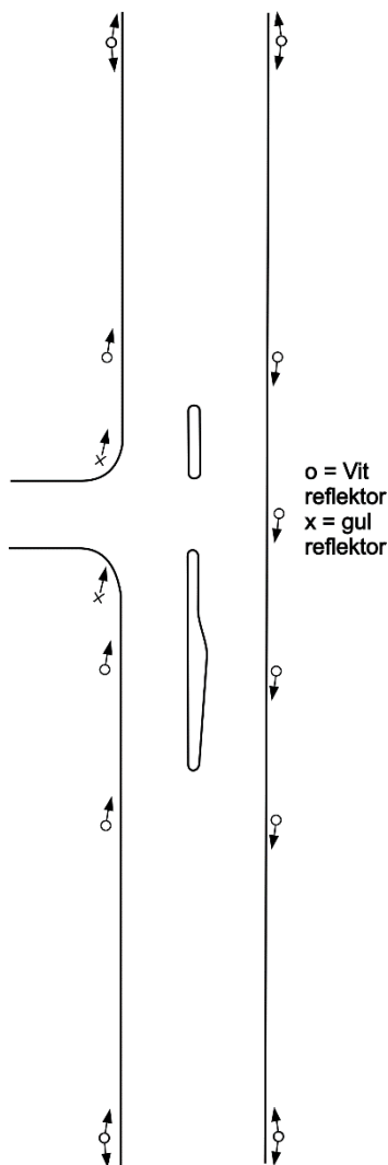
Figur 3. Placering av kantstolpar vid vägkorsning med refug. Pilarna visar retroreflektorernas riktning.
