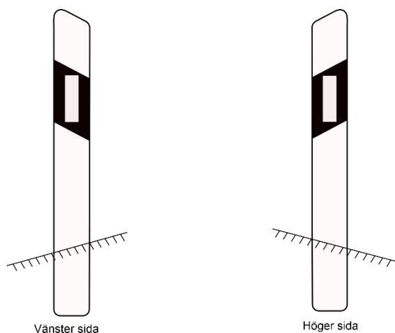
Figur 4. Kantstolpar på väg med körbana som är avsedd för trafik i endast en riktning. På stolparnas baksida ska det inte finnas någon retroreflektor.
